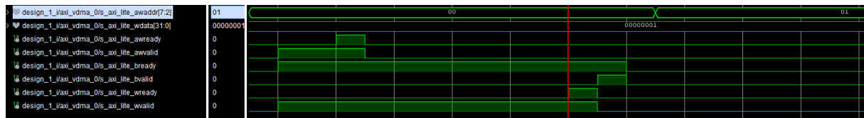
FIGURE 14 : ANALYSE SUR L'ILA DES SIGNAUX DE VDMA
